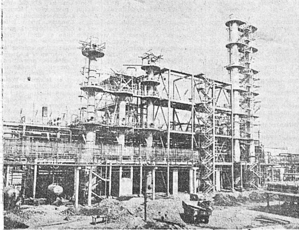
Az etilén fűzem propán-propilén szétválasztó tornyai, mellette a hozzá csatlakozó üzemrészek.
